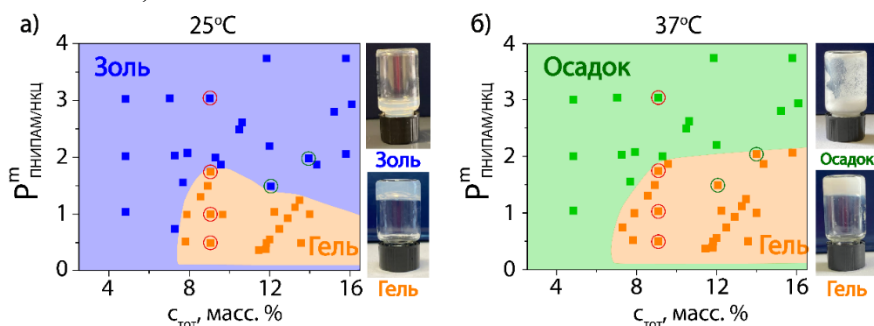
Рисунок 2 – Диаграммы состояния водной дисперсии НКЦ и ПНИПАМ при (а) 25 °C; (б) 37 °C
