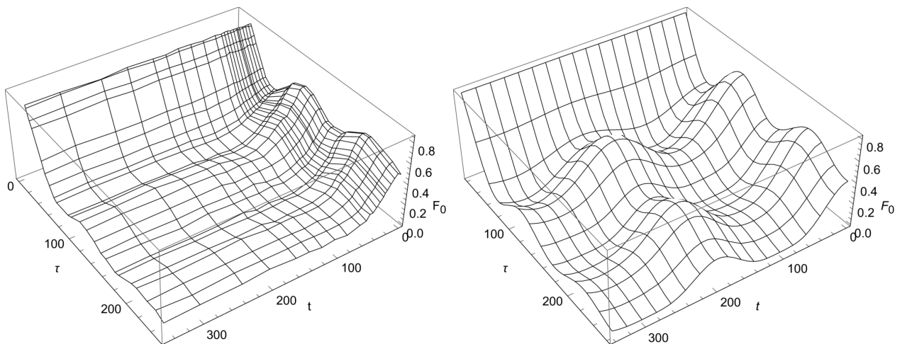
Рис. 3: Интенсивность МК когерентности порядка 0: эксперимент (слева) и теория (справа). За единицу принята интенсивность при \tau = t = 0 . \tau – длительность подготовительного периода, t – периода эволюции в микросекундах. Экспериментальные данные из работы [A2].
