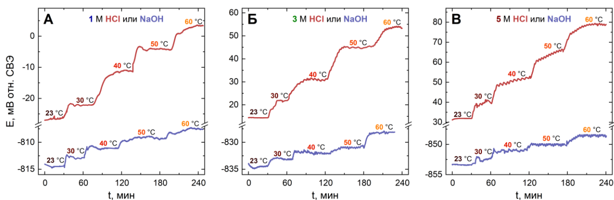
Рисунок 22 – Эволюция ПРЦ образцов ГДЭ с отдельной подачей водорода и 1, 3 или 5 М HCl или NaOH при нагреве полуячейки от 23 до 60 °С.
