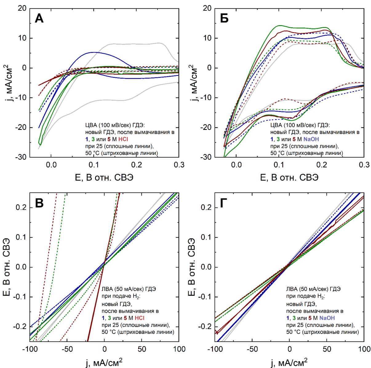
Рисунок 47 – Результаты анализа химической стабильности Pt/C в растворах HCl и NaOH: А и Б – ЦВА электродов в 1 М H 2 SO 4 в диапазоне потенциалов -0.03 – 0.8 отн. СВЭ, измеренные при 100 мВ/сек при подаче аргона; В и Г – ЛВА электродов в 1 М H 2 SO 4 , зарегистрированные в диапазоне плотности тока ±125 со скоростью развертки 50 мА/сек при непрерывной подаче водорода.
