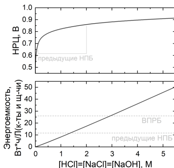
Рисунок 24 – Рассчитанные значения НРЦ и энергоемкости НПБ, использующих электролиты различной концентрации; на рисунке указаны характеристики представленных ранее НПБ и ВПРБ.
