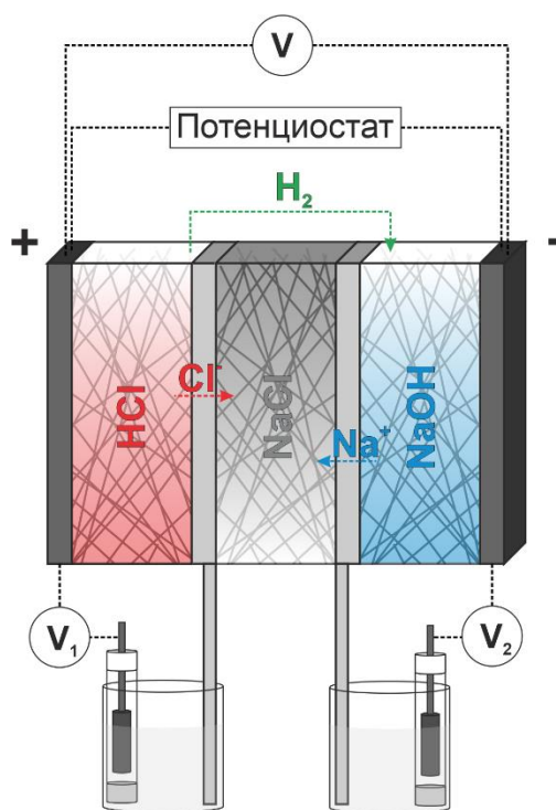
Рисунок 15 – Схема модифицированной ячейки НПБ для отдельной регистрации падений напряжения на обоих электродах.
