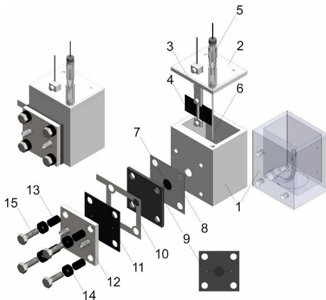
Рисунок 9 – Схема полуячейки для исследования ГДЭ: 1 – основной корпус, 2 – крышка с отверстиями для электродов, 3 – держатель противоэлектрода, 4 – противоэлектрод, 5 – ХСЭ, 6 – солевой мостик ХСЭ, 7 – образец ГДЭ, 8 – электродная прокладка ГДЭ, 9 – токосъемная пластина, 10 – токосъемник, 11 – уплотнительная прокладка, 12 – концевая пластина, 13, 14 и 15 – втулки, шайбы и болты.
