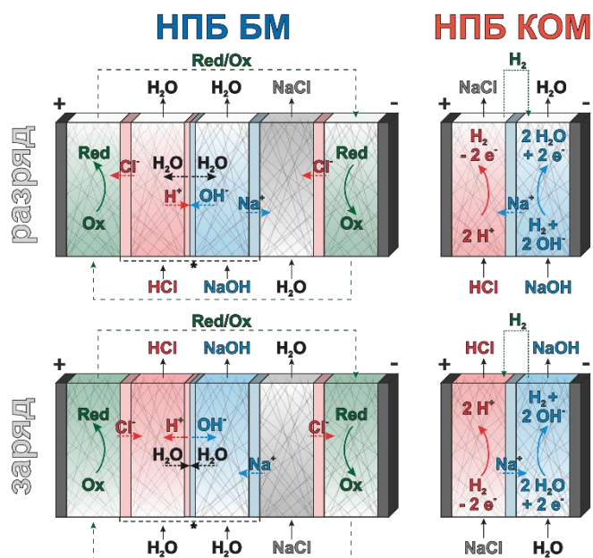
Рисунок 2 – Схема процессов, протекающих в БМ и КОМ НПБ при нейтрализации (сверху) и генерации кислоты и щелочи (снизу)
