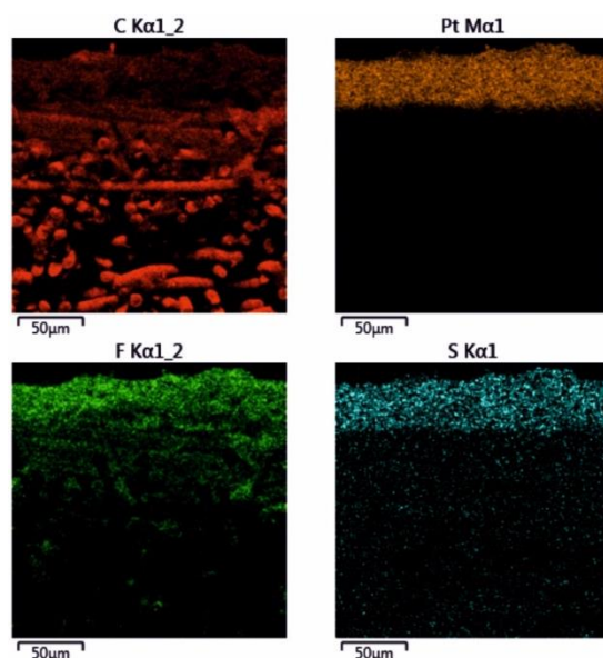
Рисунок 8 – EDX-картирование среза ГДЭ, изображенного на Рисунок 7, В по элементам С, Pt, F и S.
