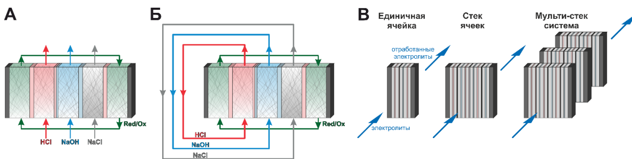
Рисунок 5 – Схема ячейки НПБ с однопроводной (А) и замкнутой (Б) системами подачи электролитов, а также масштабирования НПБ (В).
