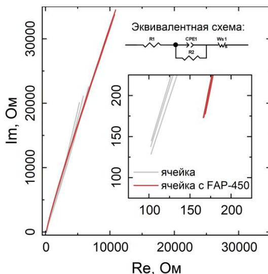
Рисунок 25 – Годографы импеданса трехэлектродной ячейки для измерения проводимости мембраны (с увеличенной высокочастотной областью спектра и указанием эквивалентной схемы для аппроксимации экспериментальных данных).
