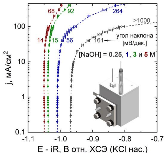
Рисунок 36 – Поляризационные кривые (с iR -компенсацией) образцов ГДЭ в условиях РОВ, контактирующих с 0.25, 1, 3 и 5 М растворами NaOH; на рисунке изображена использованная полуячейка.
