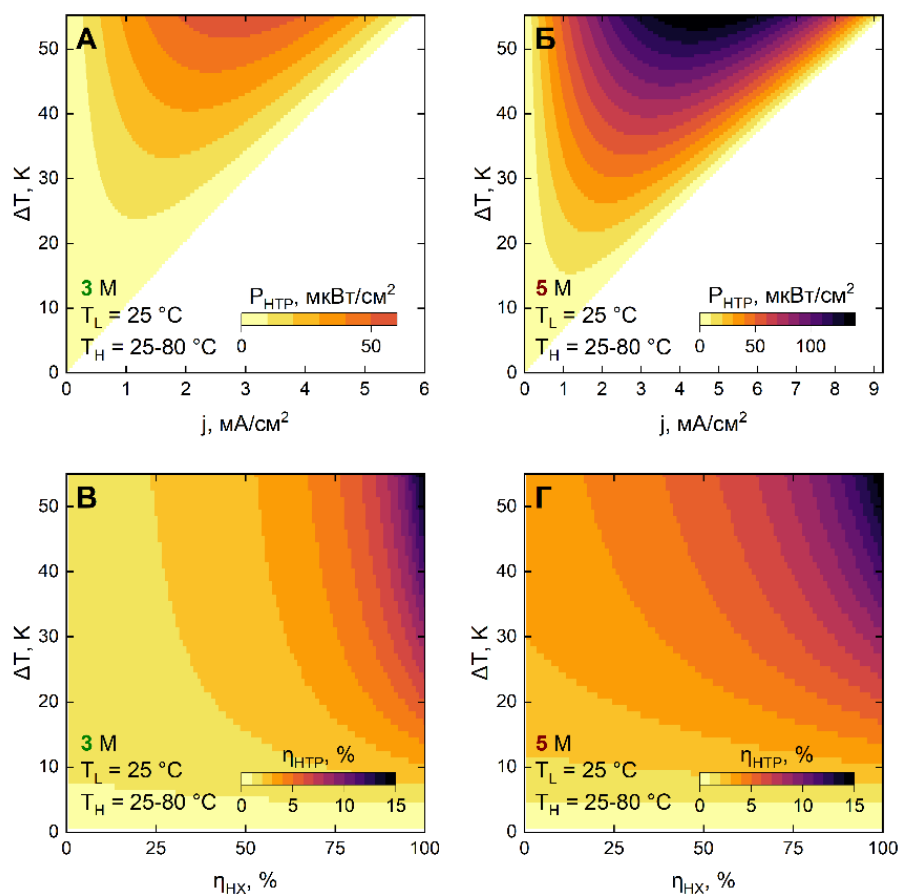
Рисунок 57 – Рассчитанные карты P_{HTP} (А, Б), и \eta_{HTP} (В, Г)
