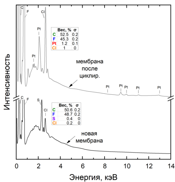
Рисунок 51 – EDX-спектры мембраны Fumaser FAP-450 до и после использования в ячейке НПБ.
