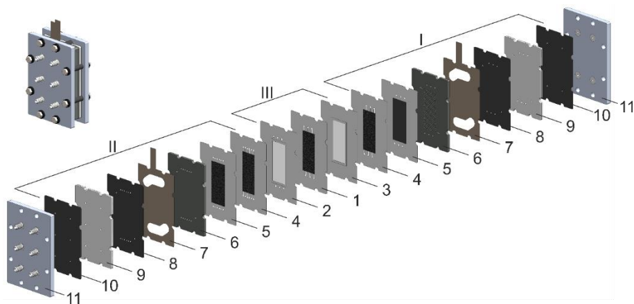
Рисунок 16 – Структура ячейки НПБ с отдельной подачей электроактивных сред на ГДЭ. Ячейка состоит из положительного (I) и отрицательного (II) полупространств и межмембранного сепаратора с АОМ и КОМ, где 1 – проточное поле с межмембранным сепаратором, 2 и 3 – прокладки с КОМ и АОМ, 4 – проточное поле с углеродной бумагой, 5 – электродные прокладки с вклеенным ГДЭ, 6 – графитовые токосъемные пластины с проточным полем для распределения водорода, 7 – металлические токосъемники, 8 – уплотнительная прокладка, 9 – прокладки проточного поля, 10 – концевая уплотнительная прокладки, 11 – концевые пластины с компрессионными фитингами.
