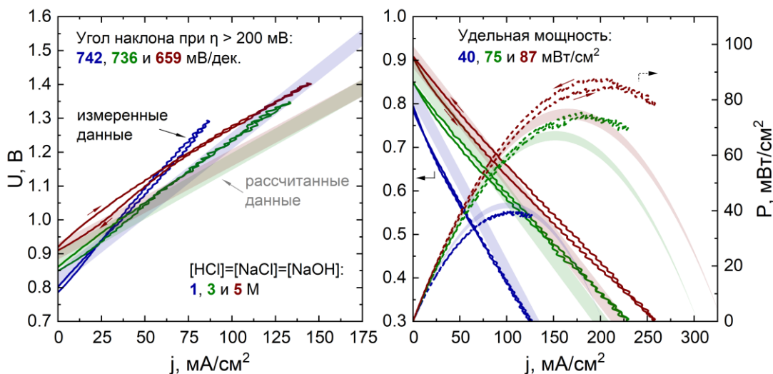
Рисунок 39 – ВАХ процессов нейтрализации (справа) и генерации кислоты и щелочи (слева) в ячейке НПБ с ГДЭ с отдельной подачей реагентов РОВ/РВВ; закрашенные кривые – измеренные данные, полупрозрачные кривые – рассчитанные данные.
