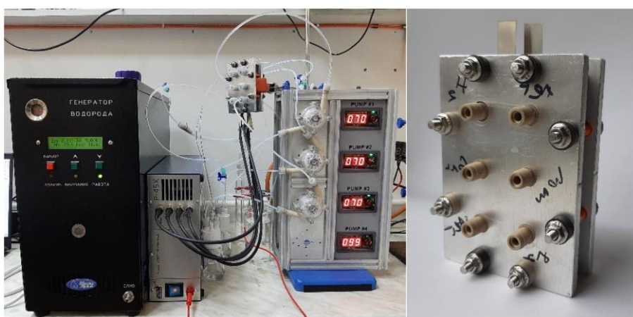
Рисунок 17 – Фотографии ячейки КОМ+АОМ НПБ (справа) и экспериментальной установки для ее исследования (слева)
