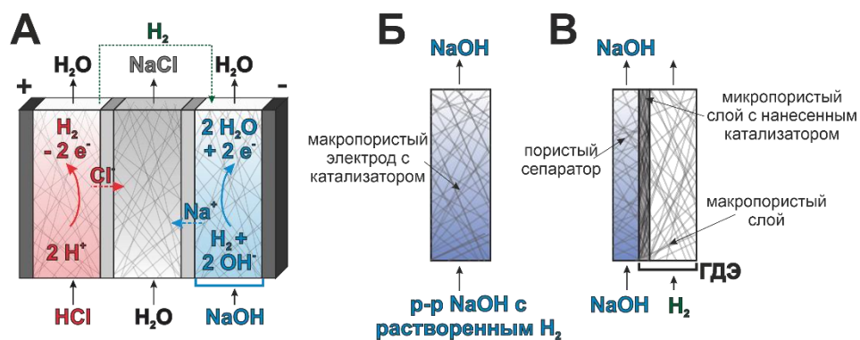
Рисунок 28 – Схема предложенной НПБ (А) с указанием смешанной (Б) и отдельной (В) подачи реагентов РОВ/РВВ на отрицательный электрод.
