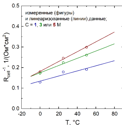
Рисунок 23 – Зависимость проводимости ячейки НПБ от температуры.
