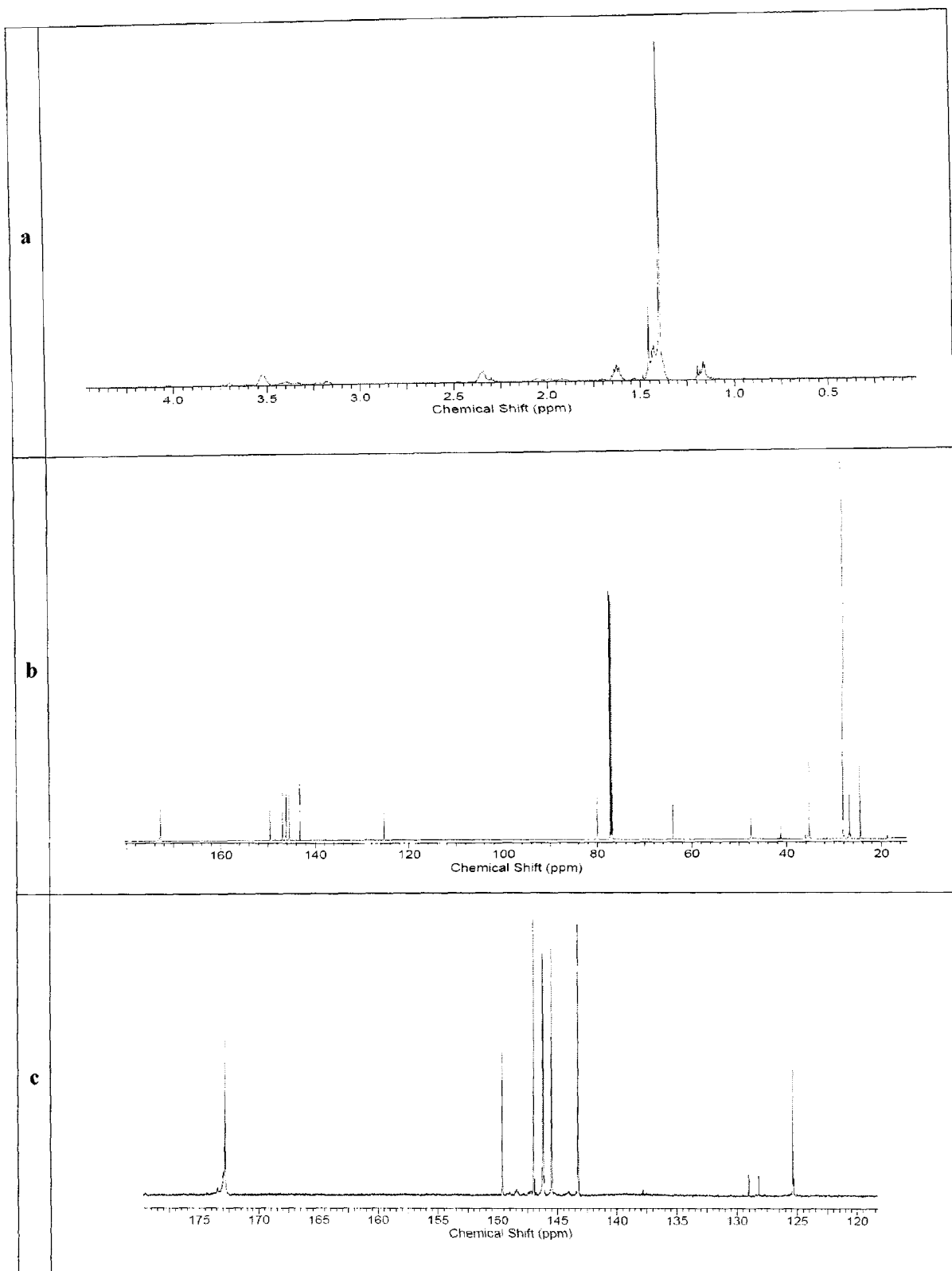
Спектр ЯМР ^1\text{H} (a), полный спектр ЯМР ^{13}\text{C} (b) и область слабых полей спектра ЯМР ^{13}\text{C} (c) аминафуллерена 3g
