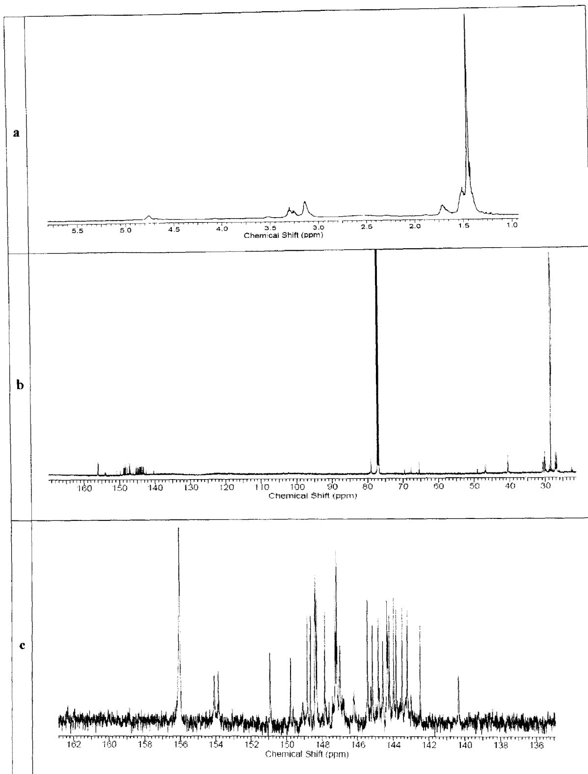
Спектр ЯМР ^1\text{H} (a), полный спектр ЯМР ^{13}\text{C} (b) и область слабых полей спектра ЯМР ^{13}\text{C} (c) аминфуллерена 3n
