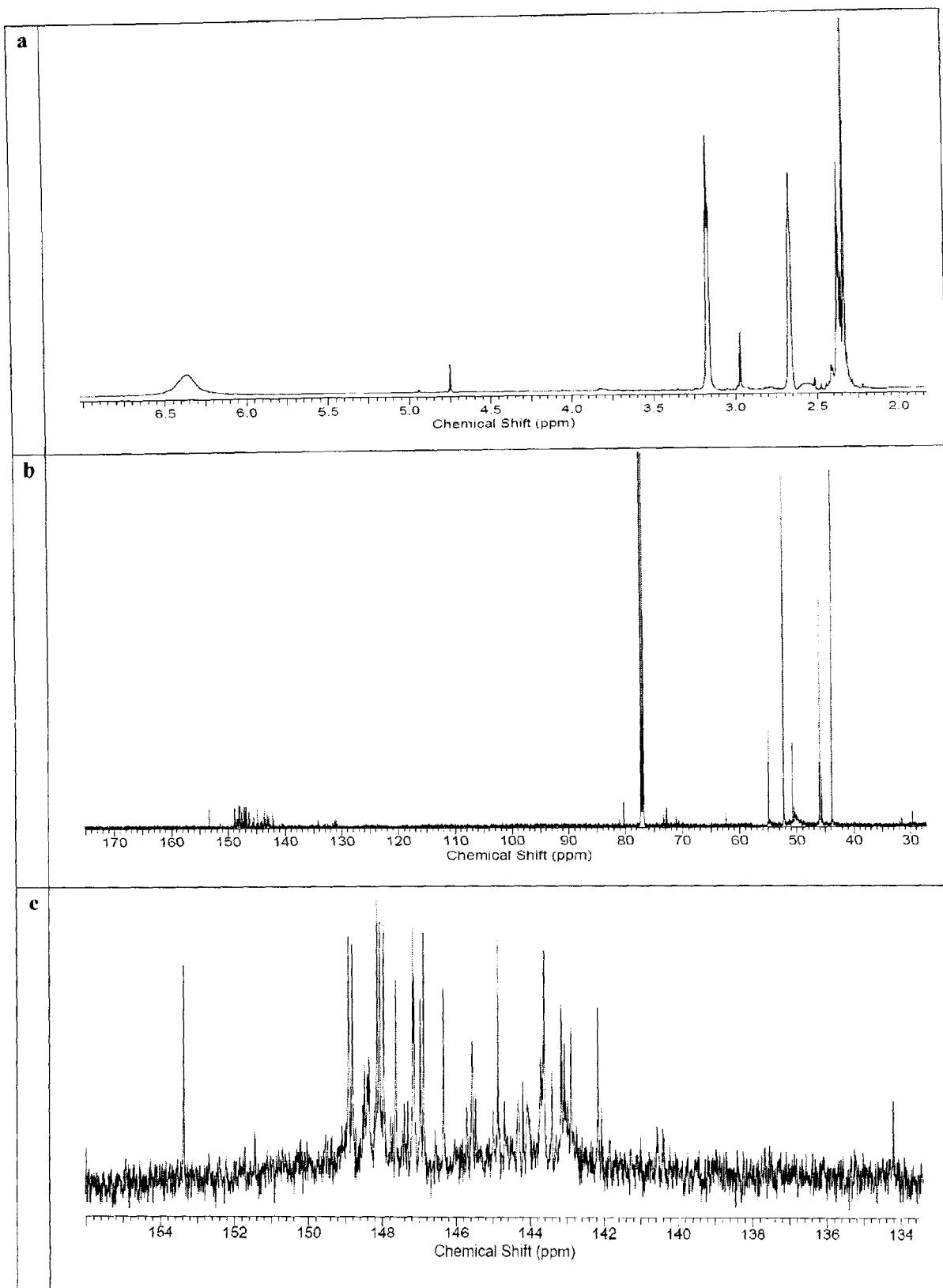
Спектр ЯМР ^1\text{H} (a), полный спектр ЯМР ^{13}\text{C} (b) и область слабых полей спектра ЯМР ^{13}\text{C} (c) аминфуллерена 3r
