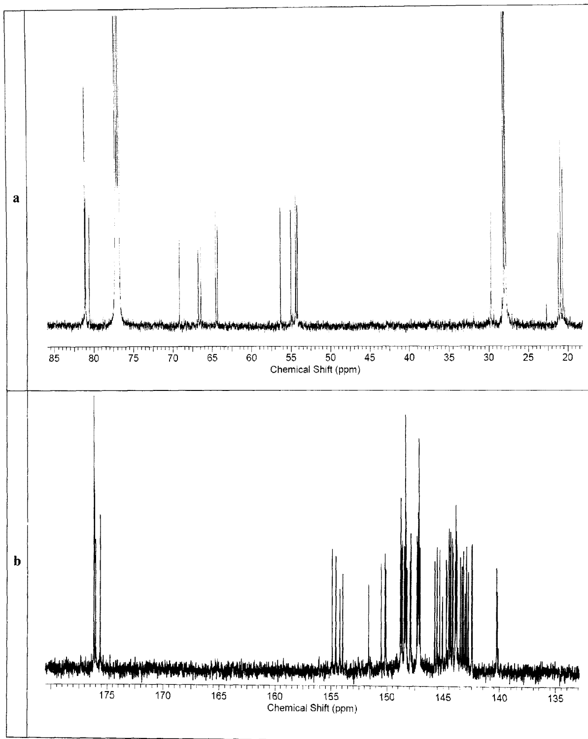
Область сильных (а) и слабых (b) полей в спектре ЯМР ^{13}\text{C} (с) аминофуллерена 3d Фиг.5
