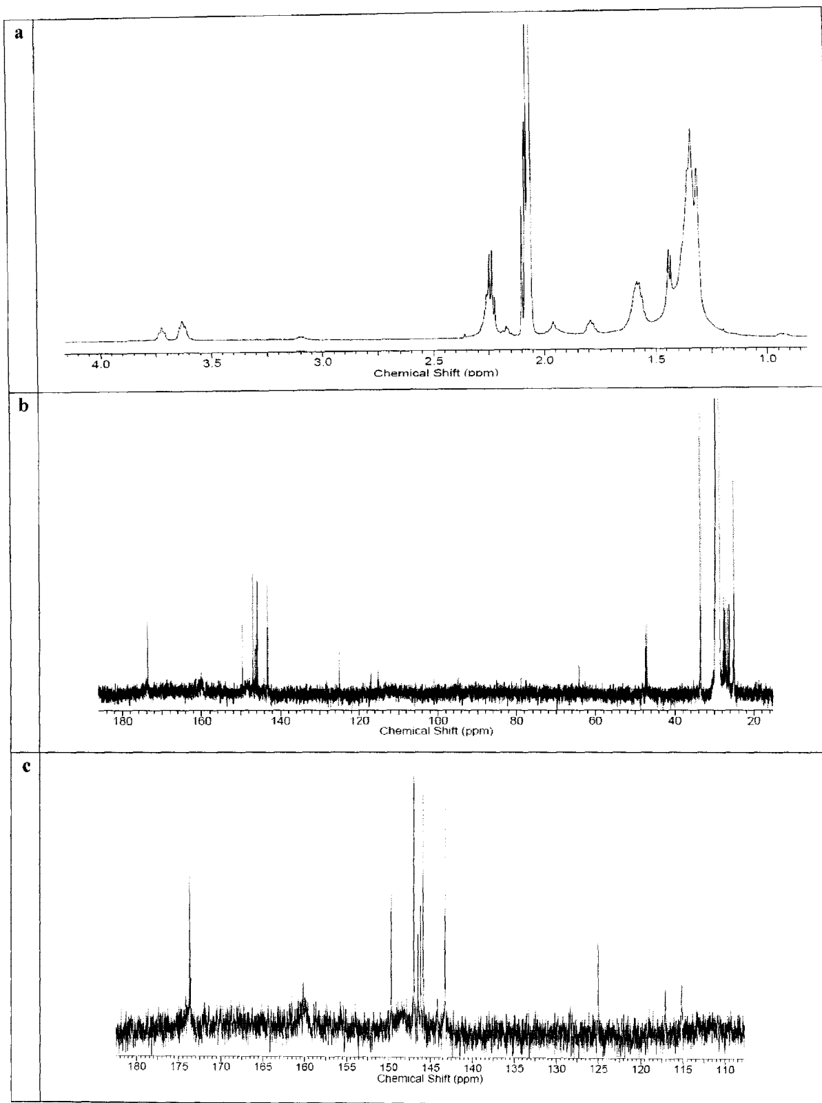
Спектр ЯМР ^1\text{H} (а), полный спектр ЯМР ^{13}\text{C} (б) и область слабых полей спектра ЯМР ^{13}\text{C} (с) аминафуллерена 3j
