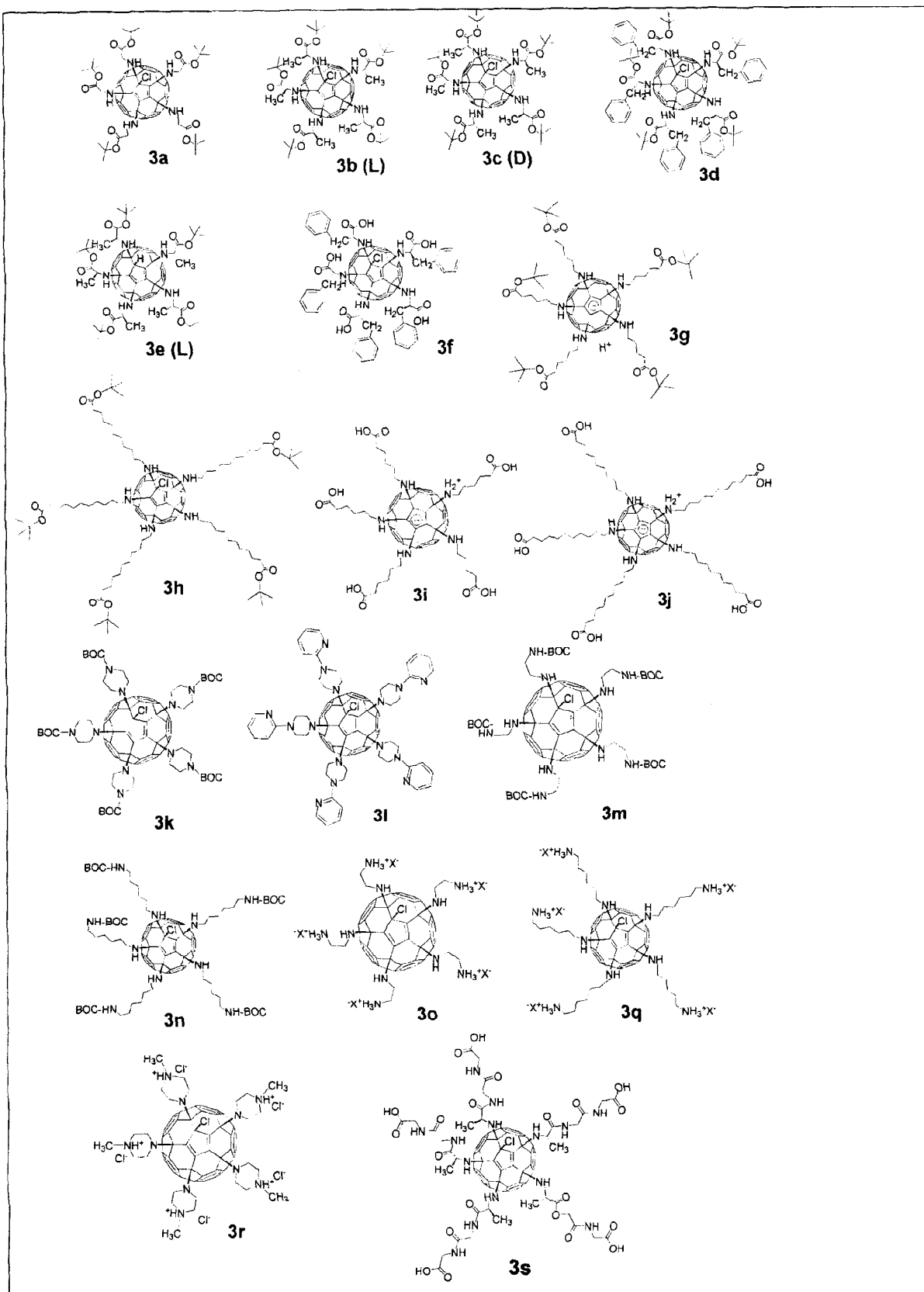
Молекулярные формулы аминфуллеренов, полученных по заявляемому способу. X = CF_3COO ; BOC = -C(O)OBu^t
