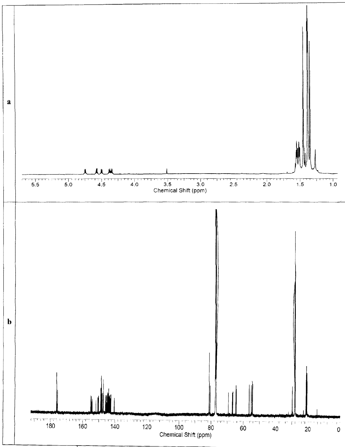
Спектр ЯМР ^1\text{H} (а) и полный спектр ЯМР ^{13}\text{C} (б) аминфуллерена 3d
